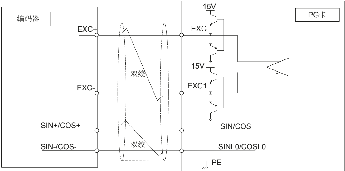
图 10-14 YD58PG4 接口回路
