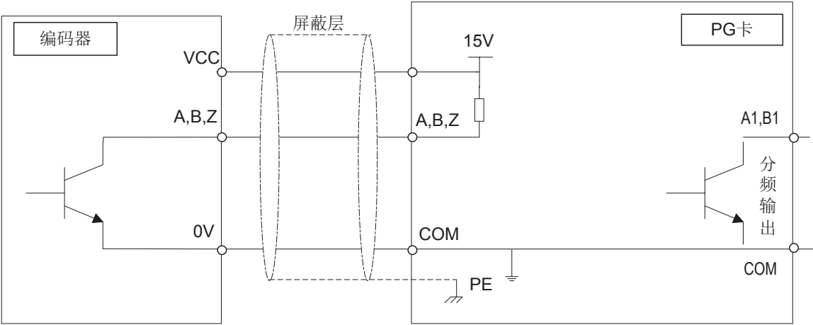
图 11-15 YD58PG5D 接口回路
