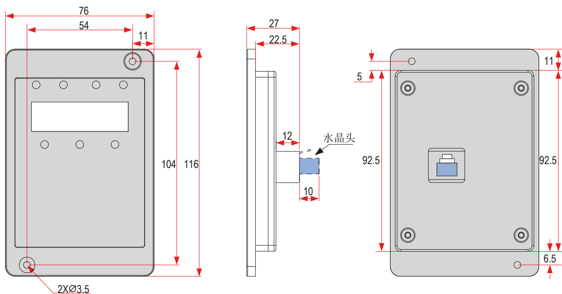
图 9-56 YD58NKE 外引操作面板尺寸（单位：mm）
