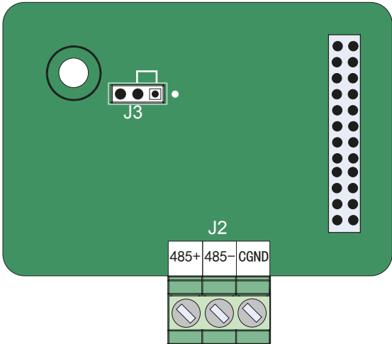
图 10-9 YD58TX1 端子分布示意图
