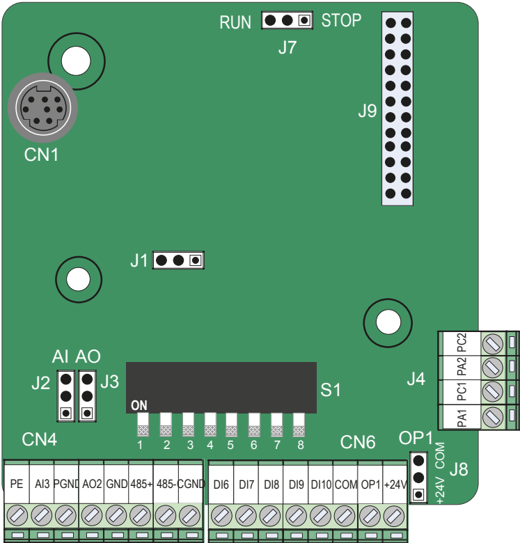
图 10-5 YD58PC1 端子分布示意图
