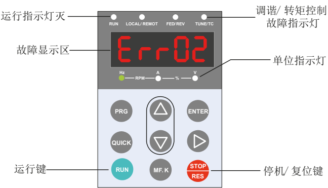
图 7-1 界面示意图
