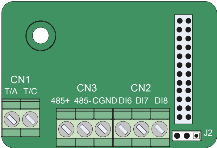
图 10-4 YD58IO3 端子分布示意图
