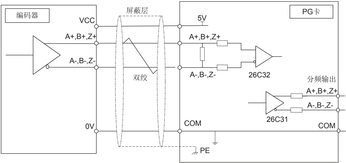
图 10-16 YD58PG6/YD58PG6D 接口回路
